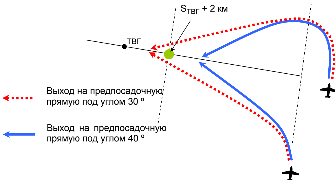
Рис. 8. Выход на предпосадочную прямую под углами 30 и 40^\circ
